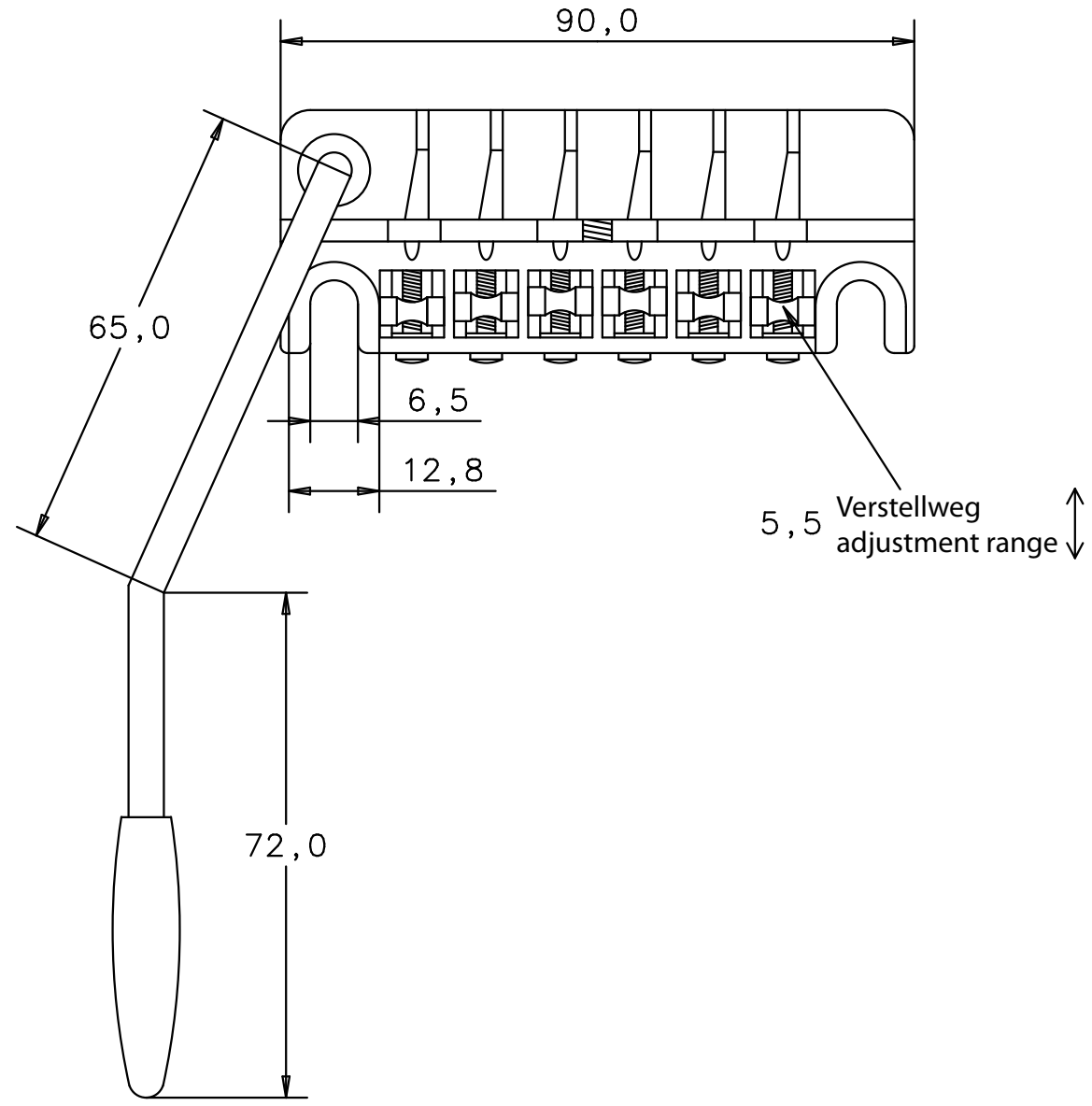
Draufsicht top view
