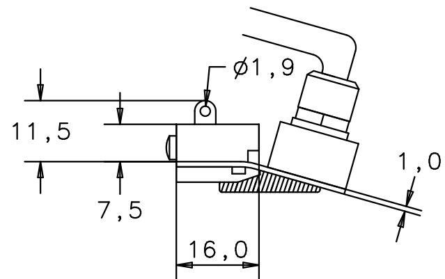
Ansicht B view B
