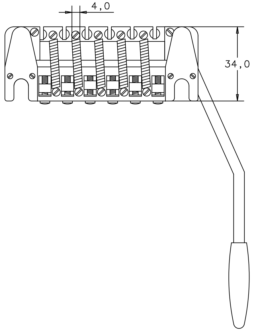
Untersicht bottom view
