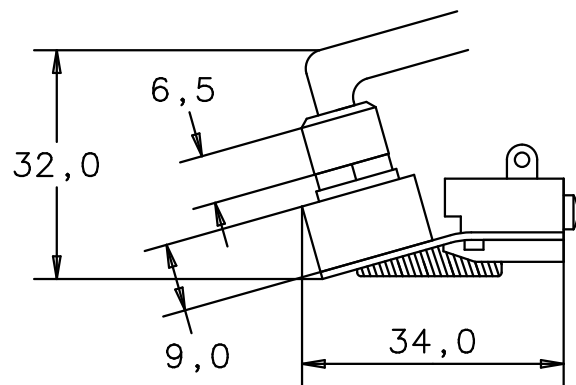
Ansicht A view A
