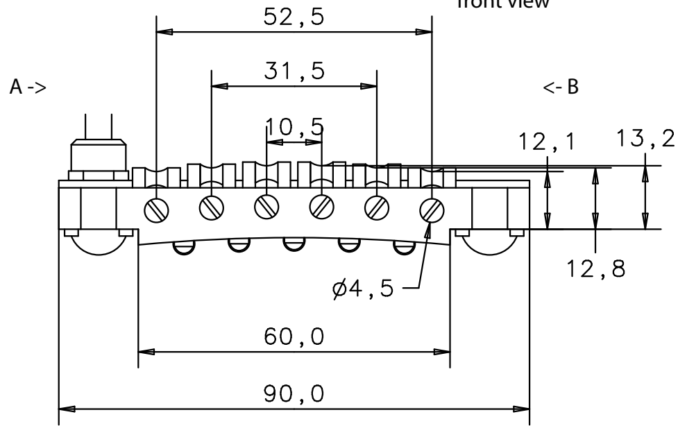
Vorderansicht front view
